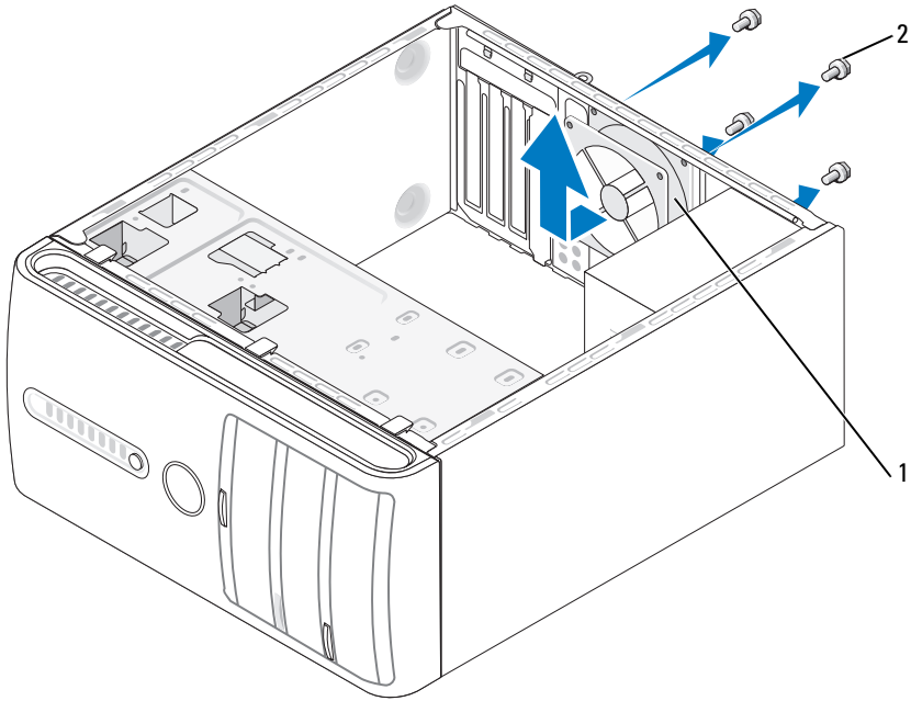
1 機箱風扇 2 螺絲 (4)
