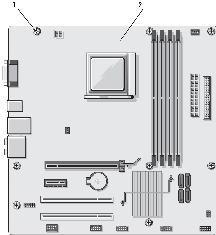
1 螺絲 (8) 2 主機板
